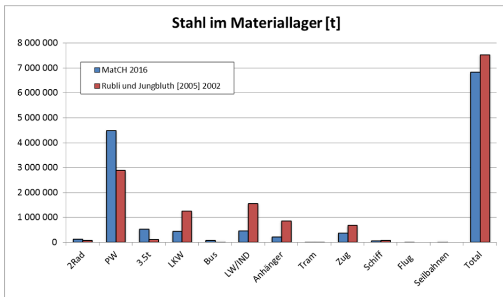
Abbildung 5-2: Vergleich Stahl im Lager (2016) mit (Rubli und Jungbluth 2005) (Zahlen 2002).
