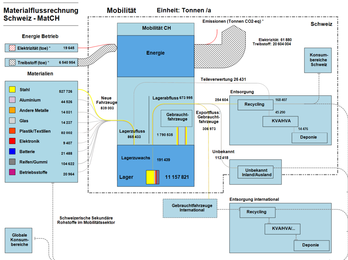
Abbildung: Übersicht der Material- und Energieflüsse im Mobilitätsbereich der Schweiz 2016.
